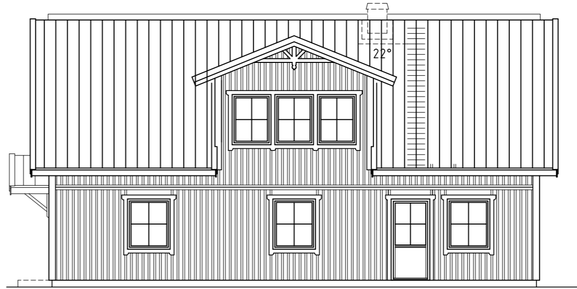
FASAD MOT
