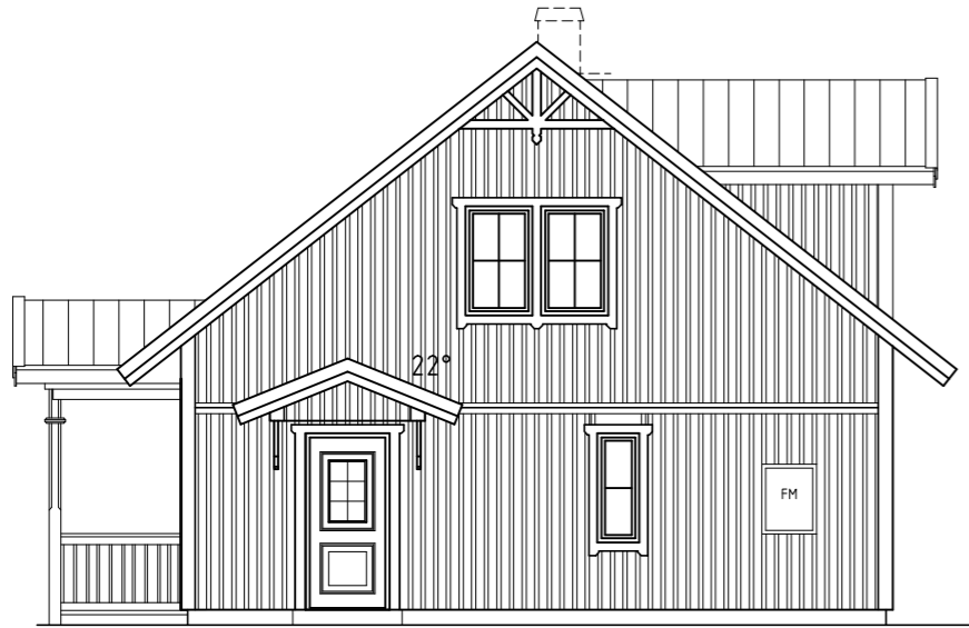
FASAD MOT
